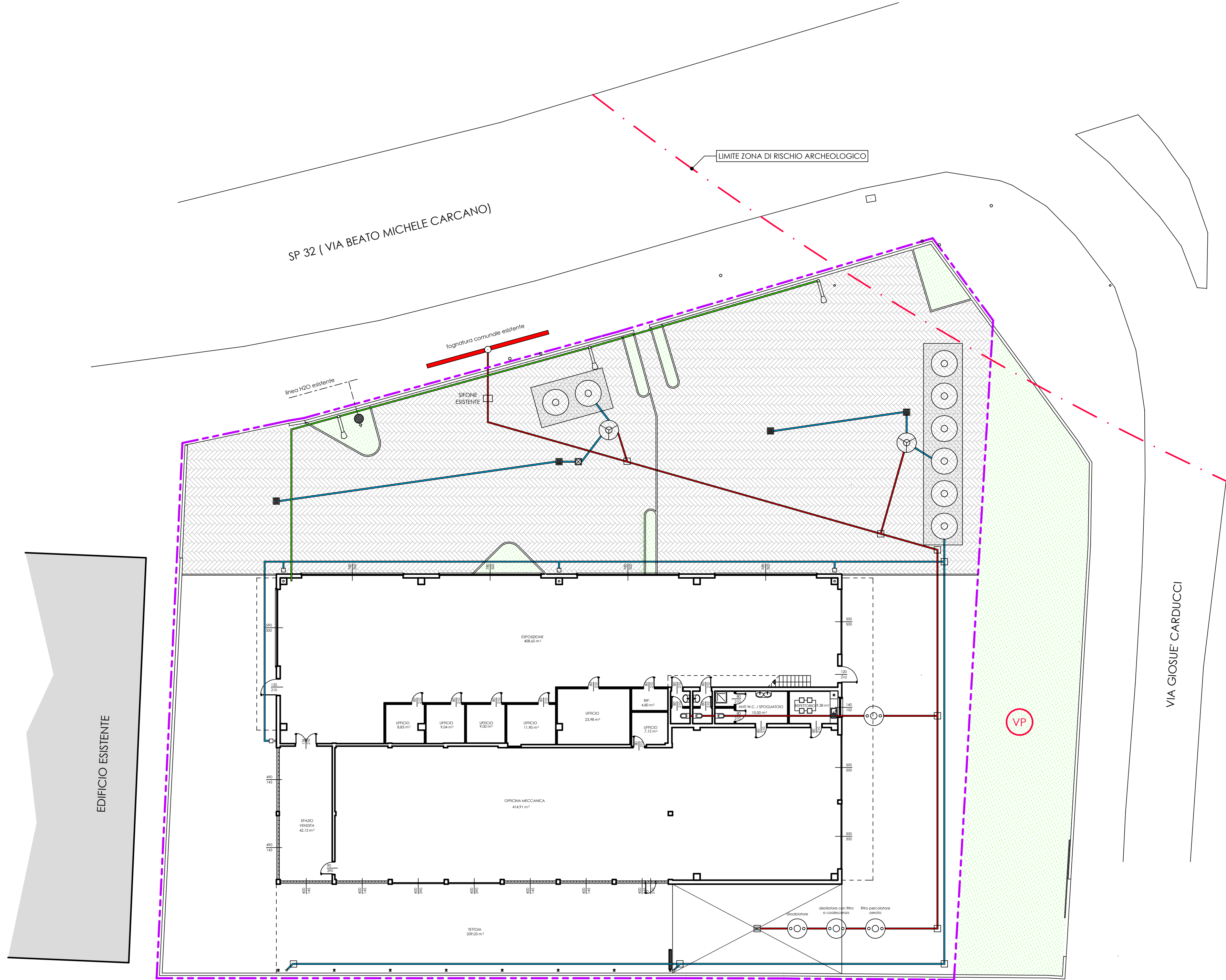
PLANIMETRIA GENERALE PIANO TERRENO
